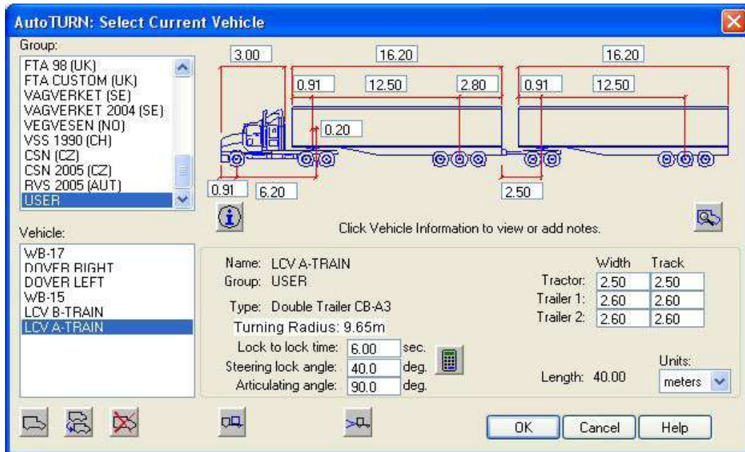
A-Train
